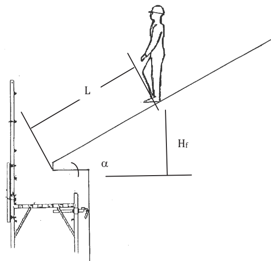
Figura 5.1.2-2 - Altezza di caduta H_f e angolo di inclinazione \alpha
