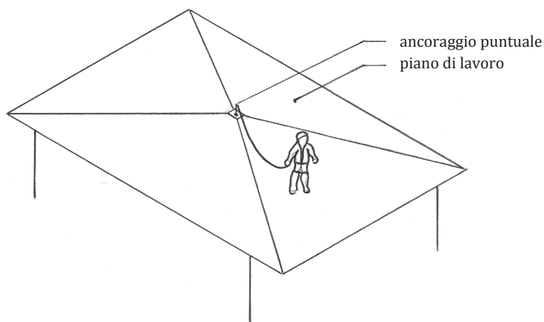
Figura 5.4.2-1 - Ancoraggio puntuale
