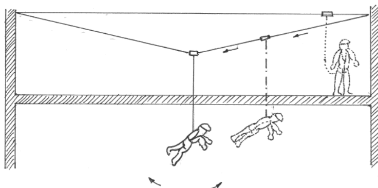
Figura 5.4.4.1-4 - Effetto pendolo su ancoraggio lineare
