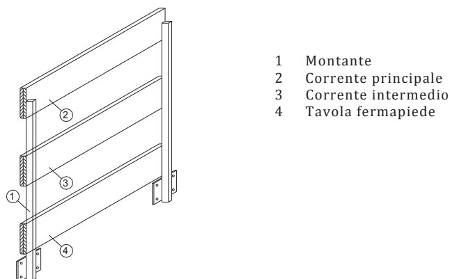
Figura 5.2.2.1-1 - Parapetto provvisorio
