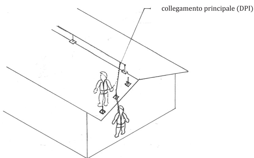
Figura 5.4.4.2-4 - Riduzione del rischio da effetto pendolo per trattenuta in caso di caduta laterale del lavoratore
