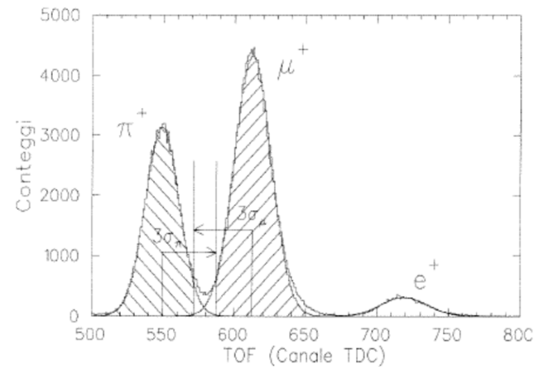
Figura 5.9: Distribuzione di TOF tra i contatori S_{-1} ed S_0 lungo un percorso di 465\text{ cm} per un fascio positivo di 146.5\text{ MeV}/c . Sono mostrati i tagli a 3\sigma operati con lo scopo di ottenere dei
