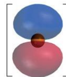
Orbitale 2p
