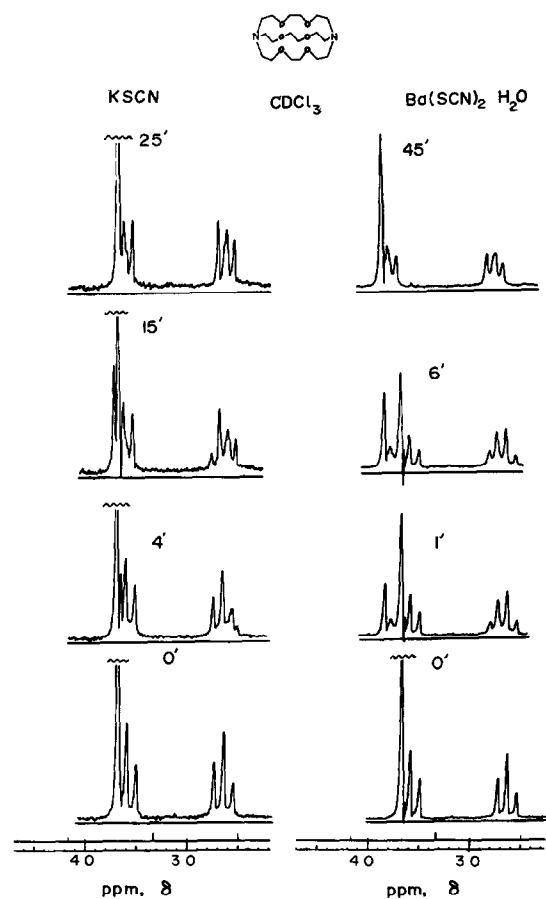
Fig 1. Observation directe par RMN (60 MHz) de la formation progressive des cryptates [2.2.2, K + ] SCN - et [2.2.2, Ba ++ ] 2SCN - à partir d'une solution du ligand [2.2.2] dans CDCl 3 et de sels solides.
