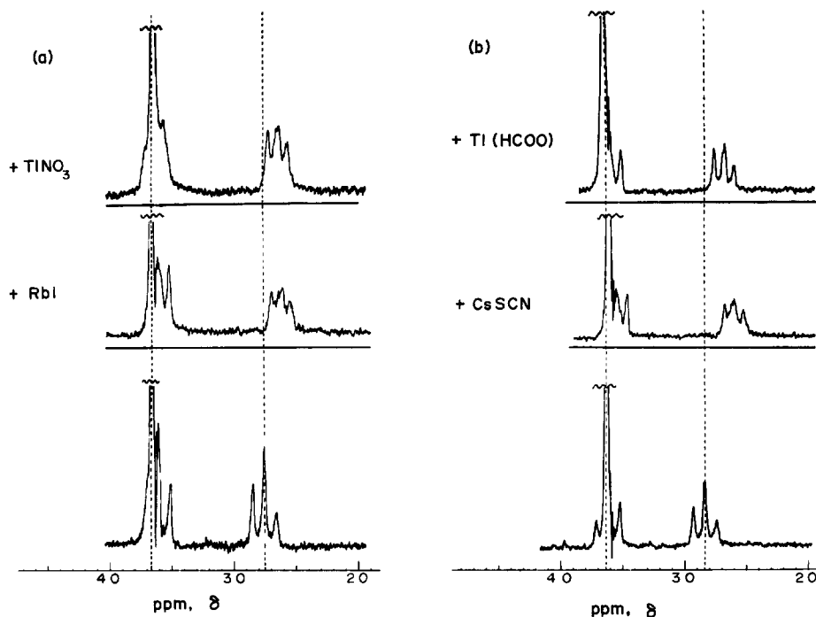
Fig 3. Spectres de RMN: (a) du ligand [3.2.2] et de ses cryptates de RbI et de \text{TiNO}_3 ; (b) du ligand [3.3.3] et de ses cryptates de CsSCN et de \text{TiOCH} (60 MHz; \text{CDCl}_3 ; TMS).
