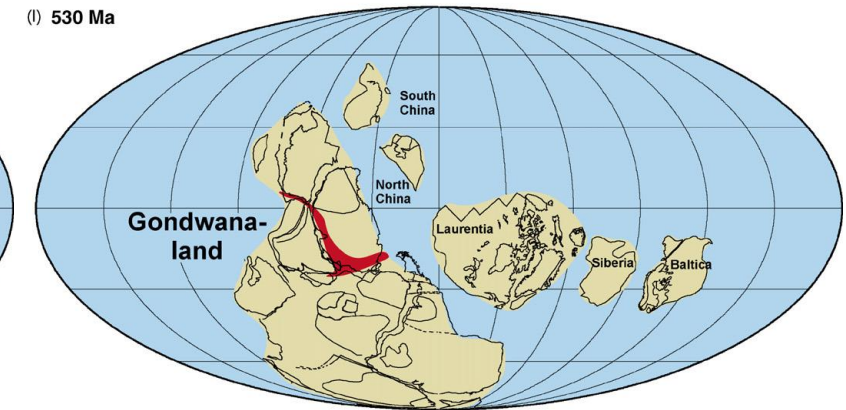
(l) 530 Ma
