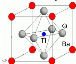
(d) BaTiO 3
