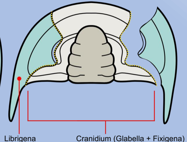
Opisthoparian
