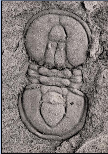
Agnostus
