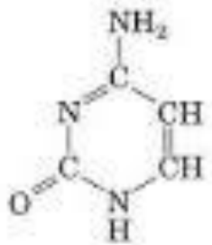
Citosina
