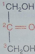
Diidrossiacetone
