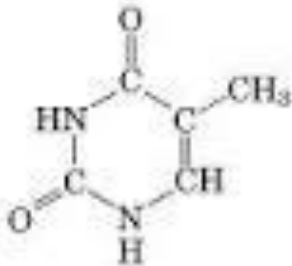
Timina (DNA)
