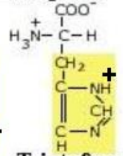
Istidina
