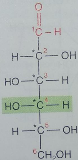
D-galattosio
