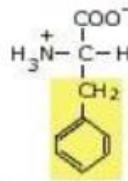
Fenilalanina
