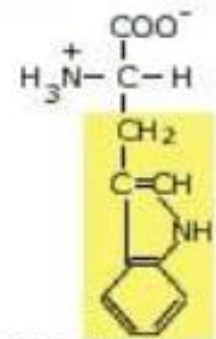
Triptofano
