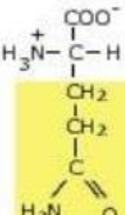
Glutammina
