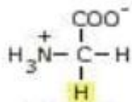
Glicina
