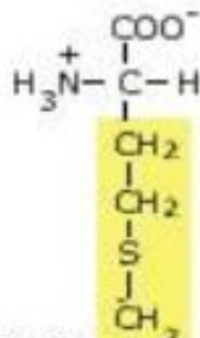
Metionina
