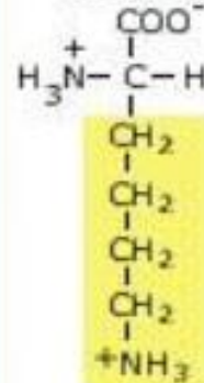
Lisina
