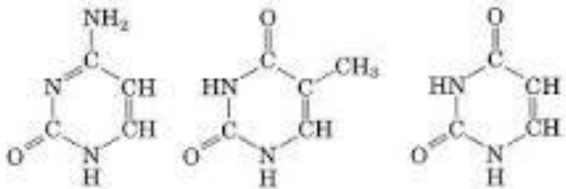
Citosina
