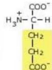
Ac. glutammico
