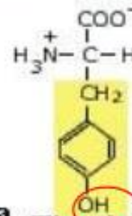
Tirosina
