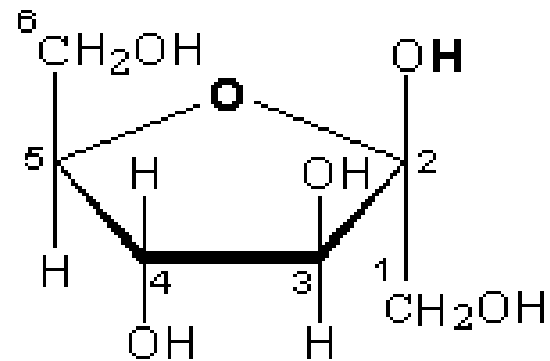
Fruttofuranosio
