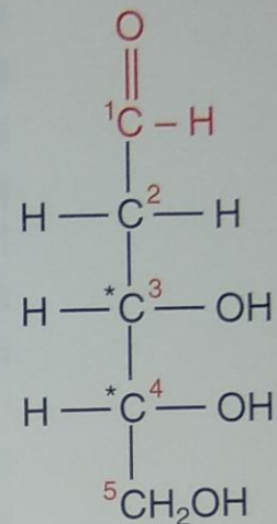
D-2-desossiribosio
