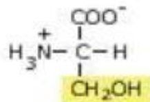
Serina
