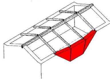
Flessione fuori piano
