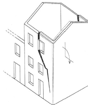
Ribaltamento timpano
