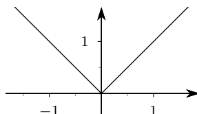
Figura 11.7 La funzione valore assoluto
