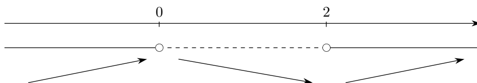
Figura 12.7 Crescenza e decrescenza di una funzione
