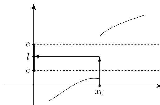
Figura 10.7 In questo caso non è possibile trovare un segmento, circondante x_0 , con le proprietà richieste
