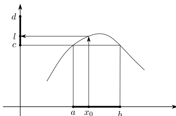
Figura 10.6 Anche in questo caso le frecce che partono dal segmento ]a, b[ cadono nel segmento ]c, d[
