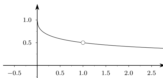
Figura 10.2 Grafico della funzione f(x) = (\sqrt{x} - 1)/(x - 1)
