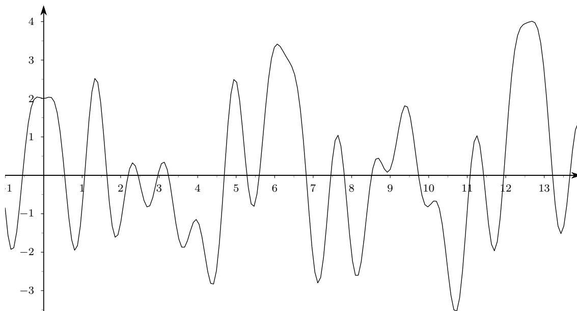
Figura 7.5 Un esempio di “funzione oscillante”
