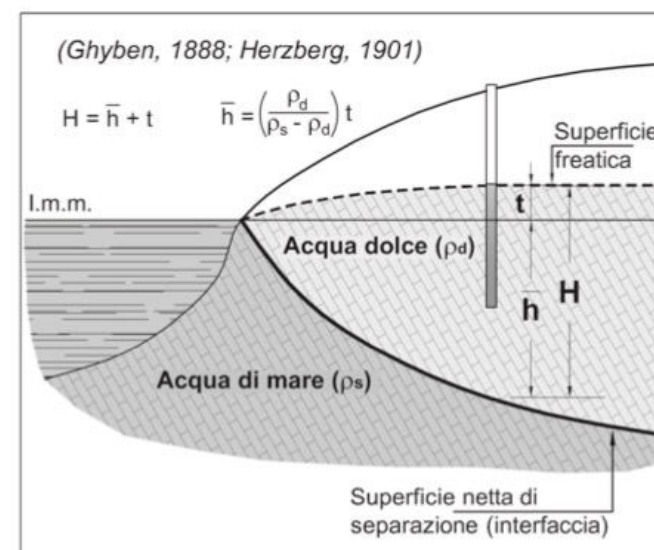
Fig. 5.2 - Condizioni di equilibrio idrostatico tra una falda di acqua dolce freatica e l'acqua di mare intrusa nel continente: relazione di Ghyben-Herzberg. Conditions of hydrostatic equilibrium between a phreatic fresh groundwater and the intruded salt-water: Ghyben-Herzberg relationship.
