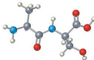
Alanilserina (Ala-Ser)
