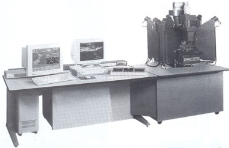
Figura 1.10 Una microsonda elettronica automatizzata fabbricata da Cameca, Courbevoie, Francia. La colonna elettronica e gli spettrometri X sono sul lato destro, il computer di controllo ed i sistemi
