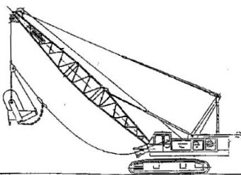
Esempio di escavatore a fune con benna per il dragaggio
