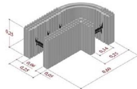
Angolo curvo
