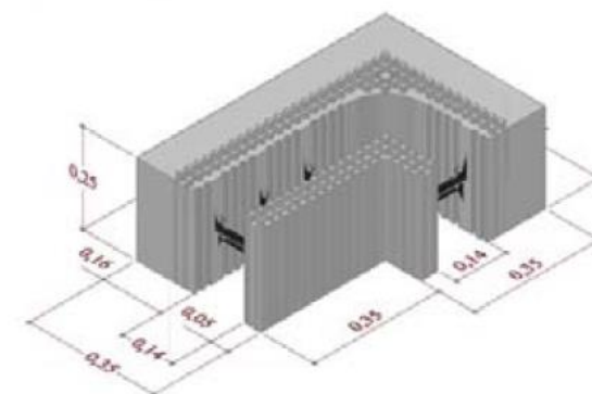
Angolo a 90°
