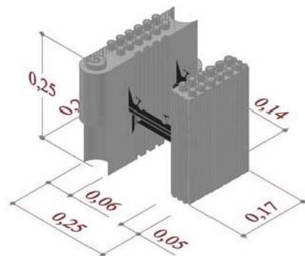
Variazione d'altezza
