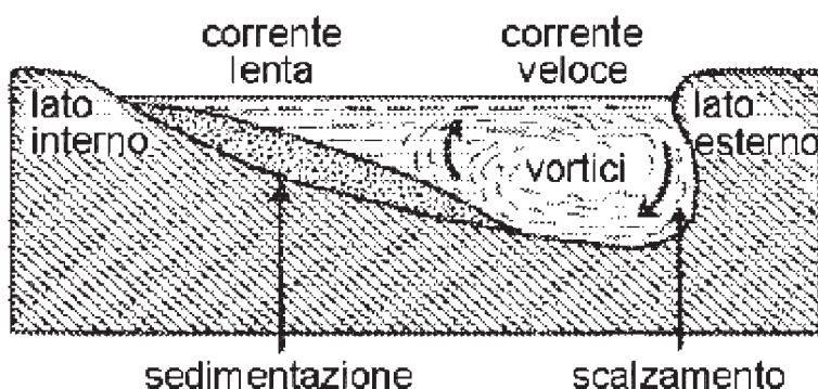
Fig. 2.13 Meccanismo di sviluppo delle anse dei meandri: erosione sulla sponda esterna e deposito su quella interna (da Money, 1977).
