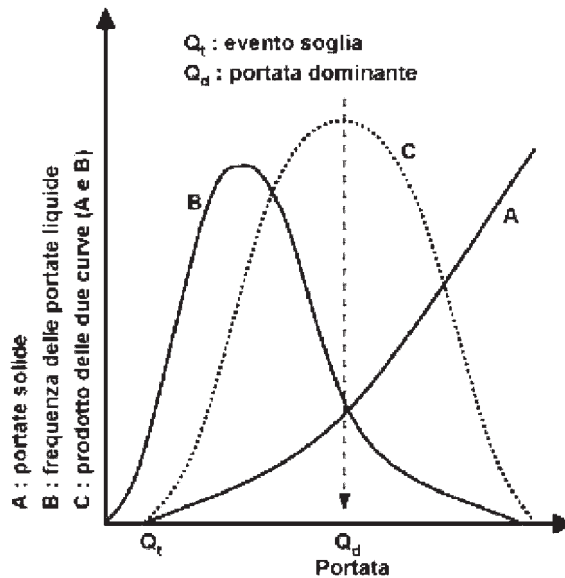
Fig. 2.10 Le portate inferiori all'evento soglia ( Q_t ) non sono in grado di effettuare un trasporto solido significativo. Portate superiori effettuano un trasporto solido crescente in maniera esponenziale (curva A), ma la loro frequenza, una volta raggiunta la moda (apice della curva B), diventa progressivamente più rara. L'apice della curva C (prodotto di A e B) corrisponde alla portata che effettua il maggior trasporto solido cumulativo nel tempo ed è detta perciò portata dominante (da Wolman e Miller, 1960).
