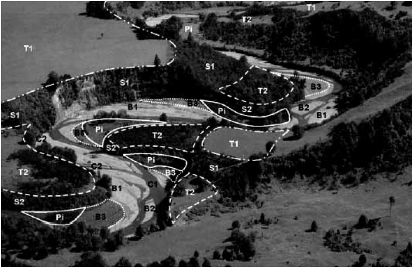
Fig. 2.8 Esempio di fiume che ha re inciso e terrazzato la piana alluvionale da esso costruita in epoche precedenti. La larghezza del solco re inciso è in stretta relazione con le dimensioni delle anse dei meandri. T1: terrazzo di primo ordine (più antico, più alto); T2: terrazzo di secondo ordine; S1 e S2: scarpate dei terrazzi; Pi: lembi di piana inondabile di recente formazione; C1 e C2: canale principale e secondario; B1, B2, B3: barre attive (laterale, longitudinale, alta) (da Franceschetti, 1980; interpretazione geomorfologica di G. Sansoni).
