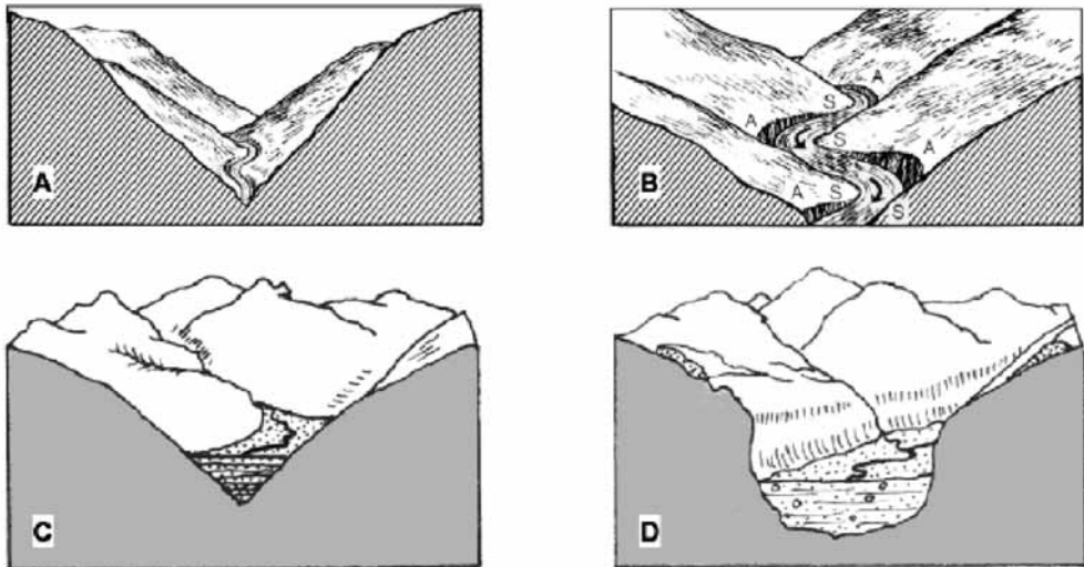
Fig. 2.6 A : Tipica valle fluviale a V. B : La stessa, incontrando rocce compatte, può iniziare a incidere sul lato esterno delle anse, formando pareti subverticali (A), alternate a speroni rocciosi (S); se l'erosione procede (ad es. a seguito di un sollevamento tettonico) si forma una forra sinuosa. C : fasi di sedimentazione possono colmare il fondo della valle fluviale. D : Tipica valle glaciale a U, col fondo colmato da depositi alluvionali. (A e B da Money, 1977; C e D da Federici e Axianias, 1981).
