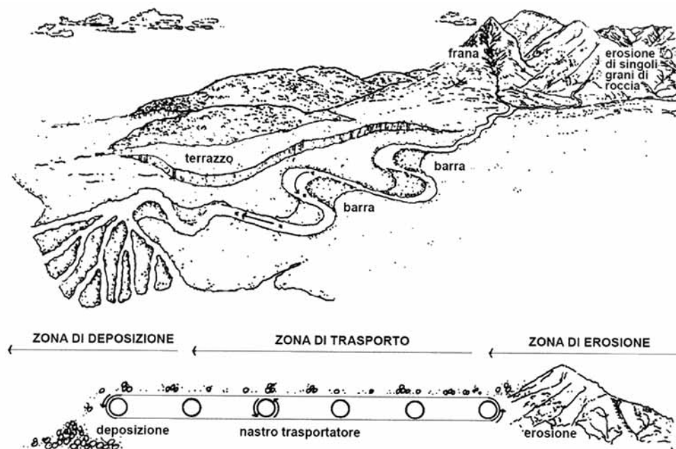
Fig. 2.9 Il corso d'acqua può essere paragonato ad un nastro trasportatore di sedimenti, dalla zona di erosione (montana) a quella di deposito (valle, lago, mare). Ciò vale sia per il corso d'acqua nel suo insieme, sia per i singoli affluenti provenienti dai sottobacini, le cui zone di erosione possono produrre sedimenti da frane, da erosione incanalata o da erosione areale e le cui zone di deposito sono rappresentate dalle conoidi di deiezione presso lo sbocco nella valle maggiore (da Kondolf, 1994, modificata nella parte montana da G. Sansoni).
