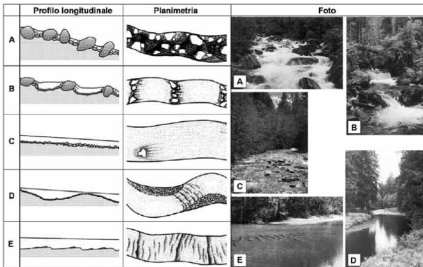
Fig. 2.16 Principali tipi di tratti fluviali. A- rapide ( cascade ); B- pozze e cascatelle ( step pool ); C- fondo piatto ( plane bed ); D- buche e raschi ( pool riffle ); E- fondo increspato ( dune ripple ) (da Montgomery e Buffington, 1997).
