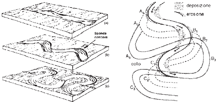
Fig. 2.14 A sinistra: ipotesi sull'origine dei meandri. (a) perturbazione trasversale del flusso da parte di irregolarità locali sul fondo o sulle rive, deviazione verso la riva opposta e inizio dell'erosione; deposito sulla sponda convessa (barra di meandro); (b) accentuazione della sinuosità: erosione e forza centrifuga si rinforzano a vicenda; (c) i meandri si allargano e migrano sia lateralmente sia verso valle). A destra: migrazione longitudinale (verso valle) e laterale dei meandri, con accentuazione della curvatura e formazione di un "collo di meandro", che verrà "tagliato" da una piena, lasciando un "ramo morto" che, isolandosi progressivamente dal fiume, diverrà una "lanca" (figura a sinistra da Hamblin, 1975; a destra da Money, 1977, modif.).
