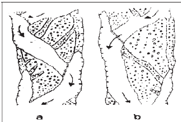
Fig. 2.12 Rappresentazione schematica dell'evoluzione e della migrazione di un canale a bassa sinuosità (da Billi, 1988).
