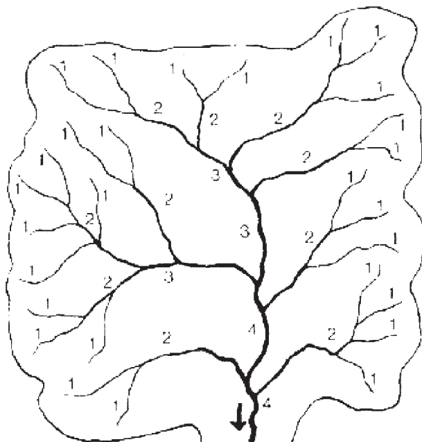
Fig. 2.5 Ordinamento gerarchico di Strahler dei rami di un reticolo idrografico (da Money, 1977).
