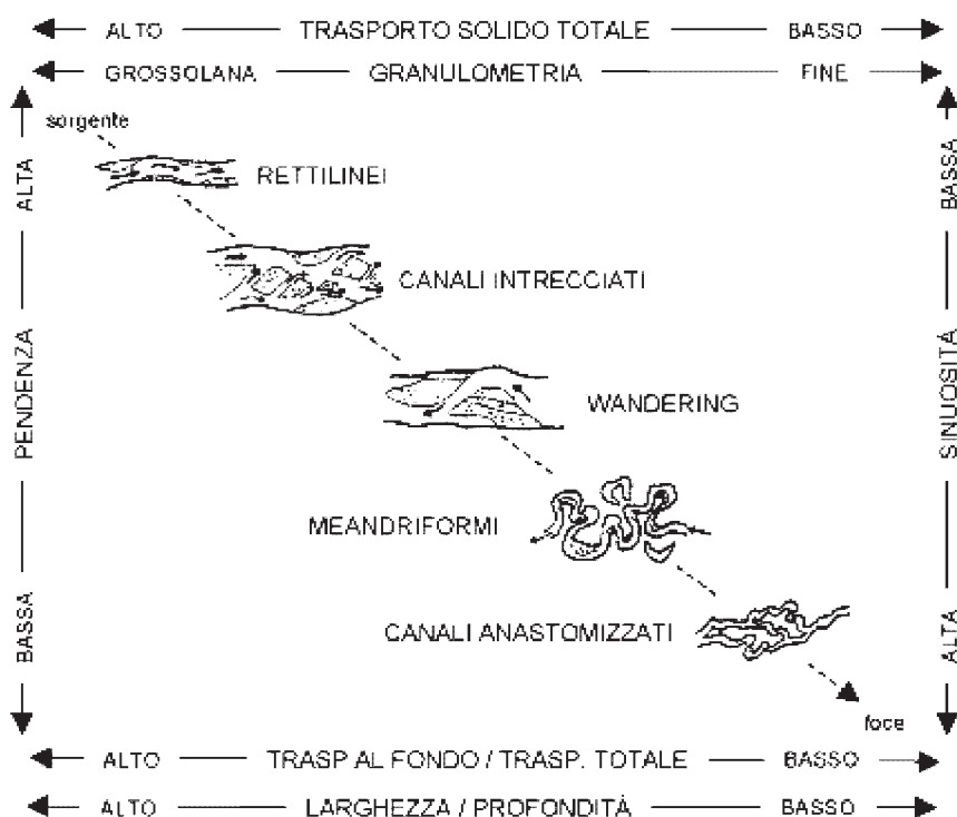
Fig. 2.11 Classificazione schematica delle principali morfologie d'alveo, con l'indicazione sommaria dei parametri che le condizionano maggiormente. Sebbene nella figura le configurazioni siano ordinate dai tratti montani a quelli di pianura, nella realtà alcune di esse possono essere assenti e i casi reali possono presentare diverse anomalie (da Billi, 1988, modif.).
