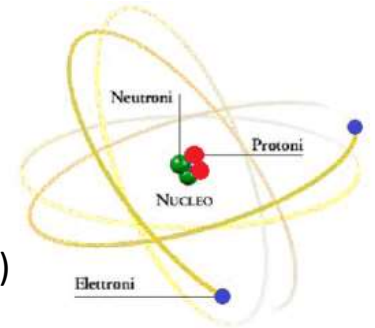
Struttura atomica della materia
