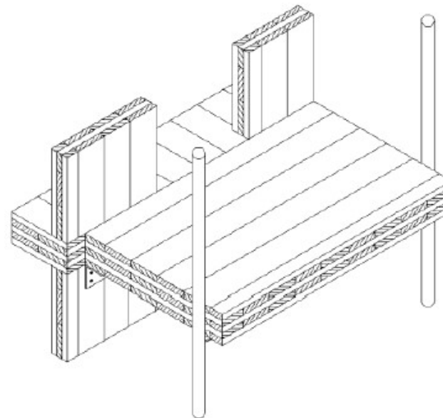
Pannello XLAM appoggiato su staffe metalliche fissate alla parete e su pilastri esterni
