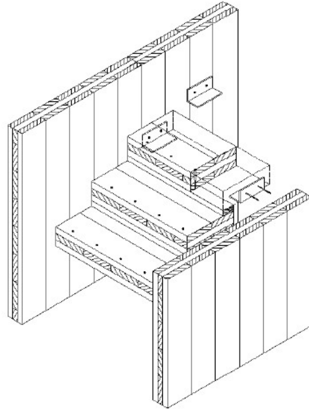
Gradini collegati alle pareti mediante angolari metallici avvitati
