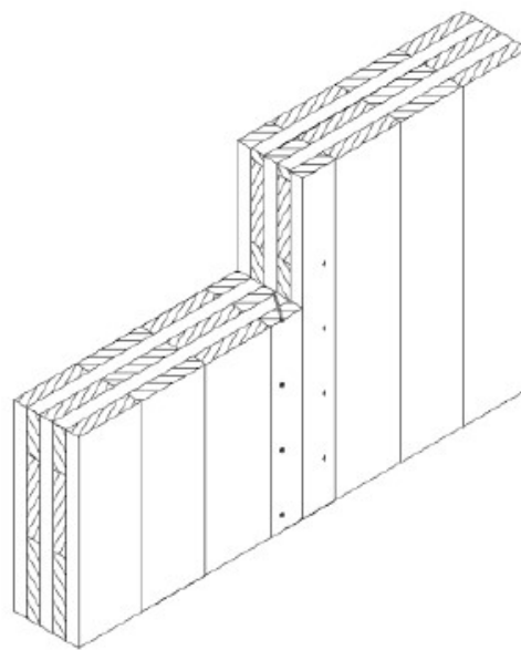
Giunto con viti incrociate
