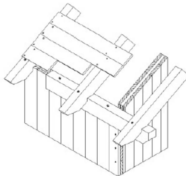
Copertura a travetti
