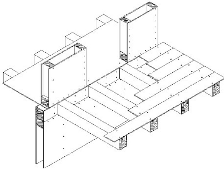
Travi balcone in continuità con quelle del solaio
