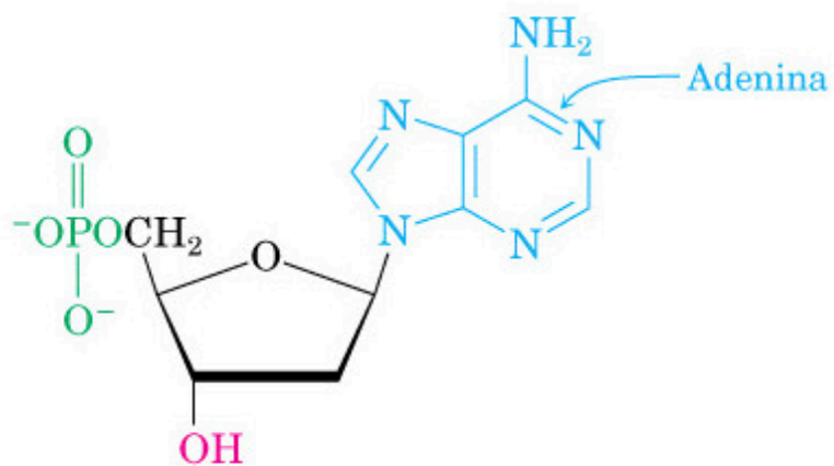
2'-Deossiadenosina 5'-fosfato
