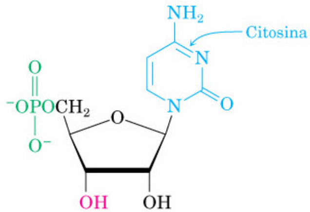
Citidina 5'-fosfato
