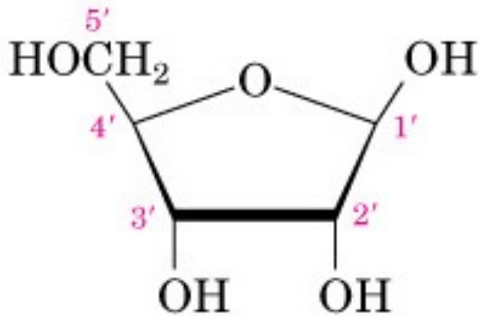
Ribosio
