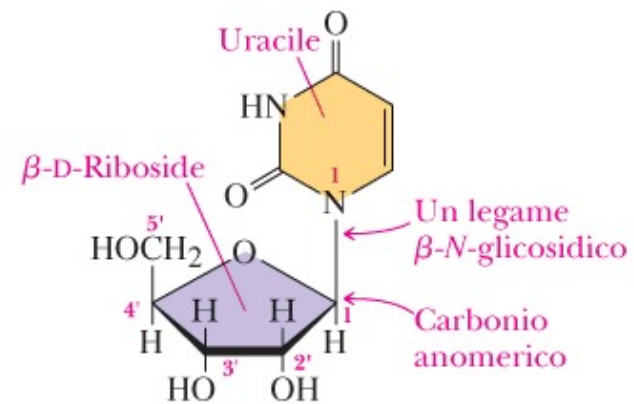
Uridina
