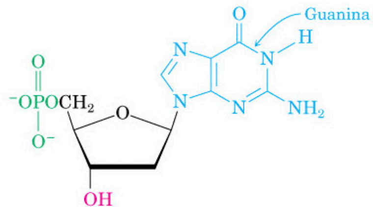
2'-Deossiguanosina 5'-fosfato
