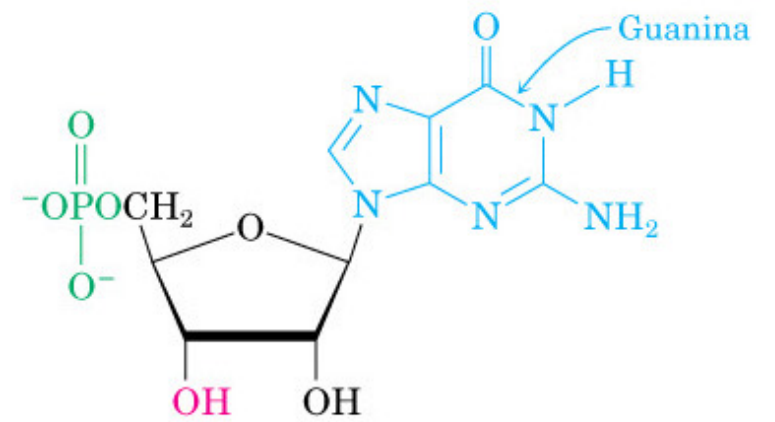
Guanosina 5'-fosfato
