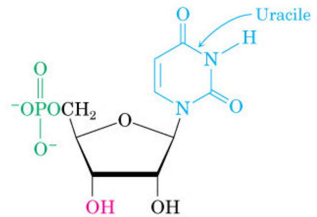
Uridina 5'-fosfato
