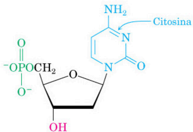
2'-Deossicitidina 5'-fosfato
