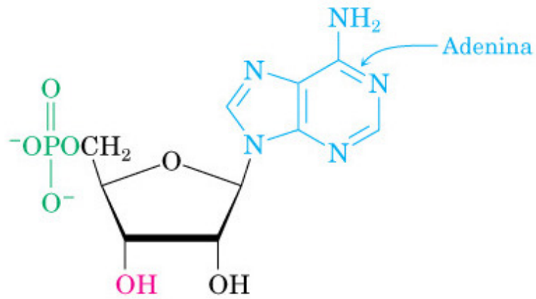
Adenosina 5'-fosfato
