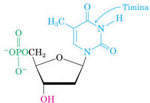
2'-Deossitimidina 5'-fosfato
