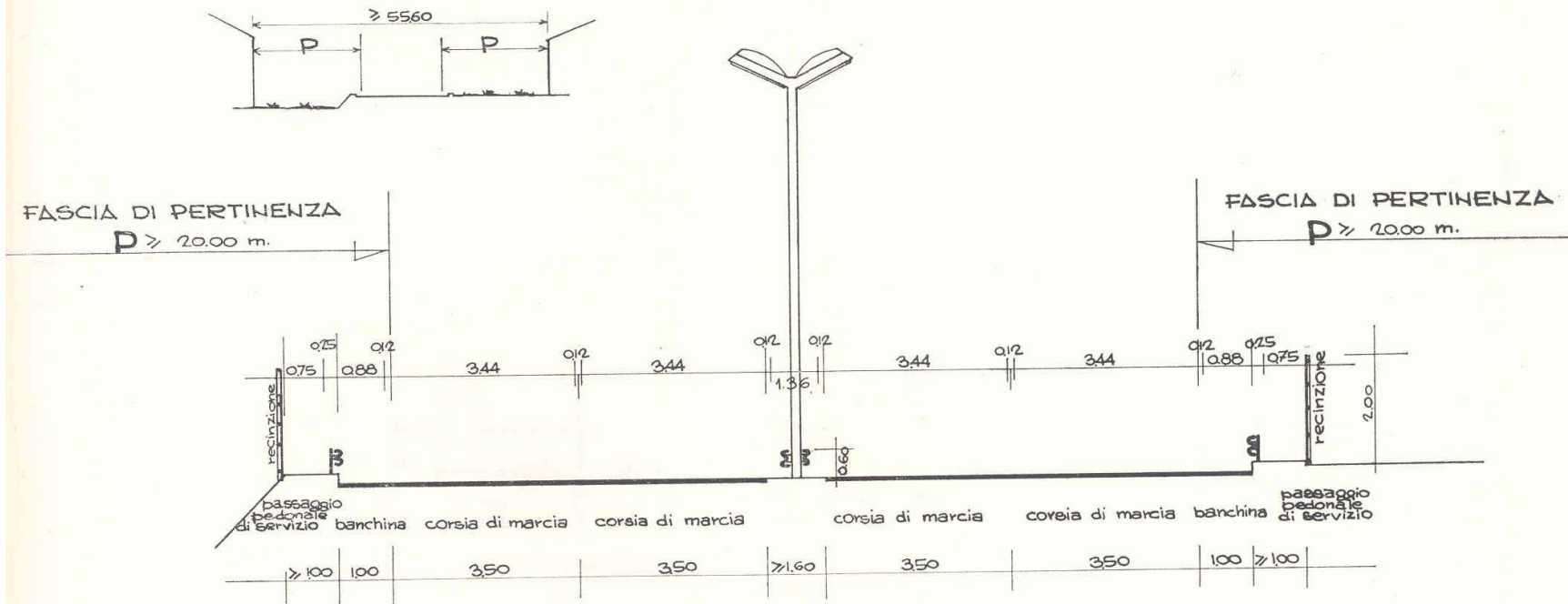
Fig. 5 - STRADA PRIMARIA TIPO: sezione corrente a 2 corsie/senso (cat. 1.a).
