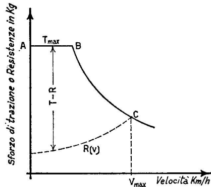
FIG. II.17 - Caratteristica di trazione (trattore a potenza costante).
