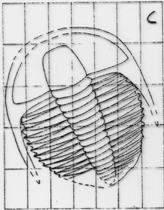
FIG. 3.66 DEFORMAZIONE DI FOSSILI. C = STATO INDEFORMATO DA RAULSAY E HUBER, 1984
