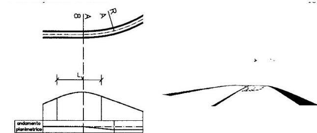
Fig.3 - Curva planimetrica mascherata da un dosso [8]
