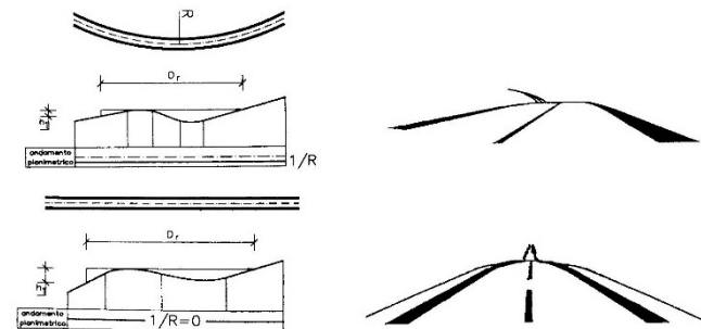
Fig.8 - Esempi di perdita di tracciato. Con h_i è indicata l'altezza dell'occhio del conducente [8]
