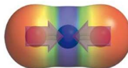
26 Diossido di carbonio, \text{CO}_2
