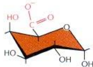
\alpha -D-Galacturonic acid (GalA)
