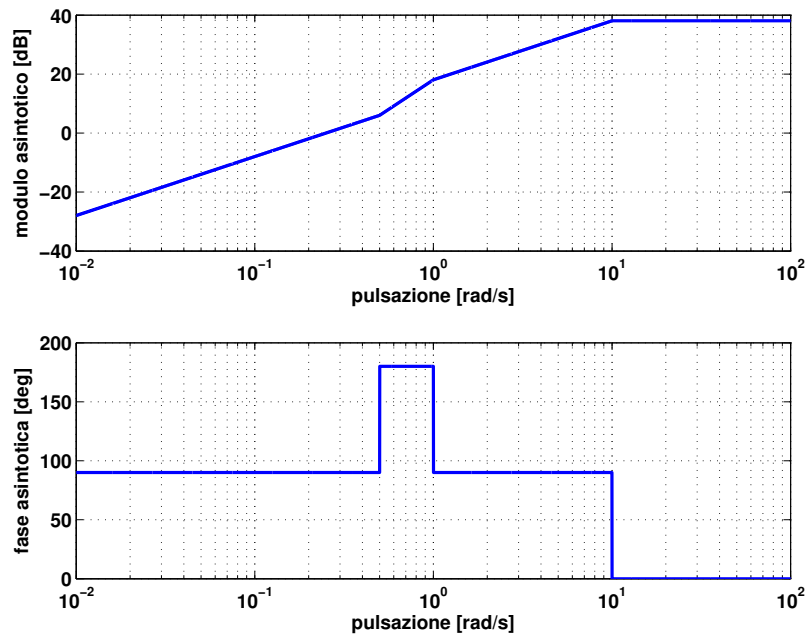
Figura 1: Diagramma di Bode asintotico
