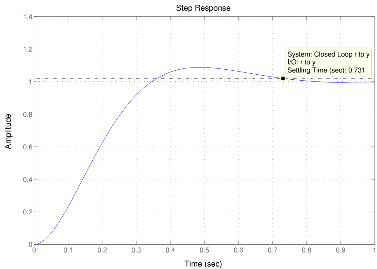
Figura 5: Risposta allo scalino a ciclo chiuso, con in evidenza il tempo di assestamento.
