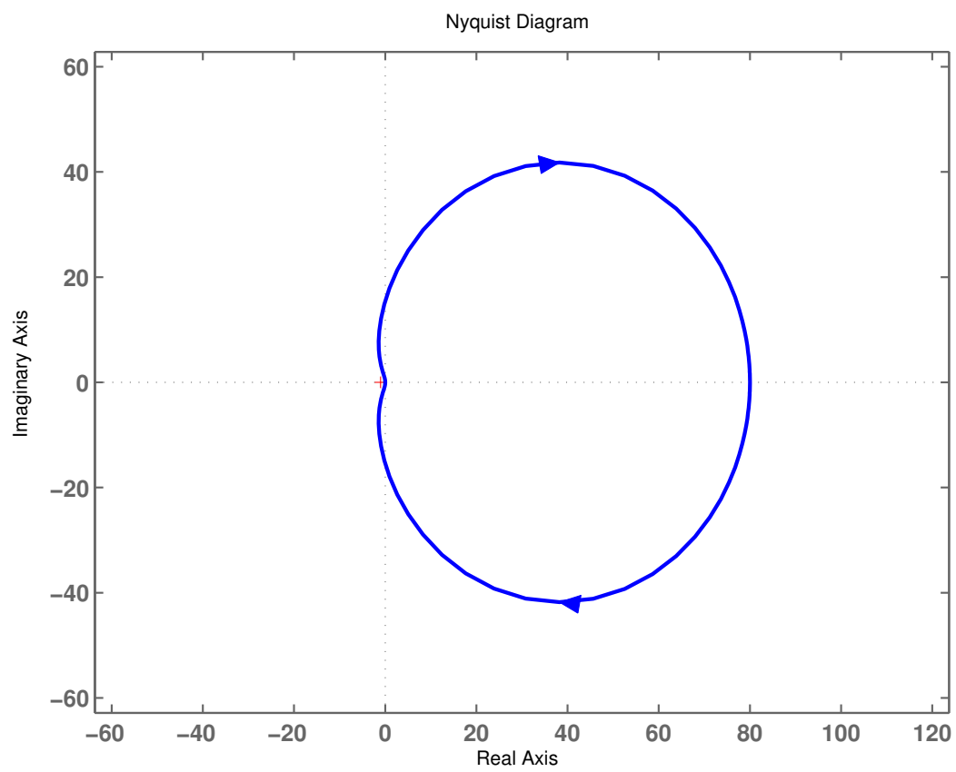
Figura 2: Diagramma di Nyquist della Fdt L(s) .
