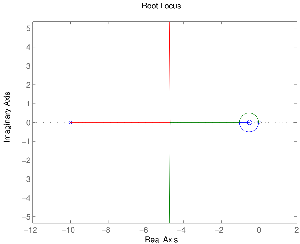
Figura 7: Luogo delle radici cercato. I diversi colori individuano come si muovono le radici sul luogo al variare del guadagno k .
