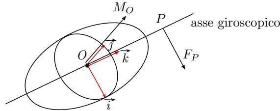
Figura 13.6.6: Effetti giroscopici
