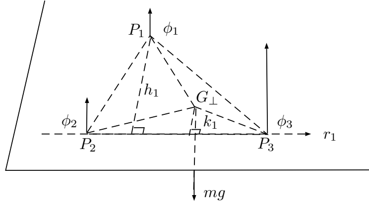
Figura 13.1.1: Treppiede
