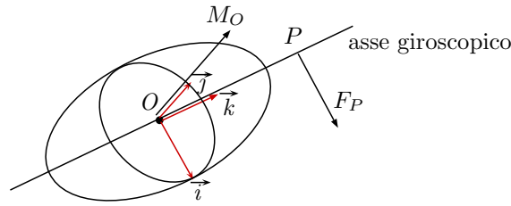
Figura 13.6.2: Giroscopio
