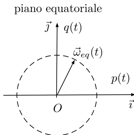
Figura 13.6.3: Componente equatoriale della velocità angolare
