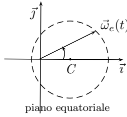
Figura 13.6.7: Componente equatoriale della velocità angolare
