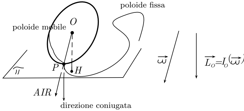
Figura 13.6.5: Moto alla Poincot
