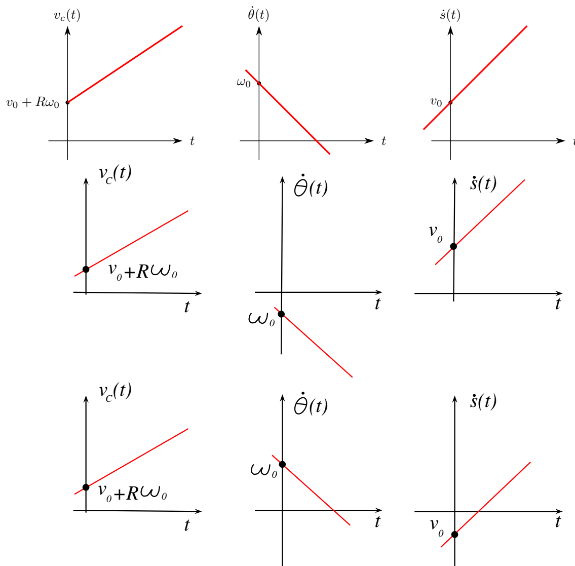
Figura 13.7.1: Disco su guida di grande inclinazione, con velocità iniziale di strisciamento positiva.
