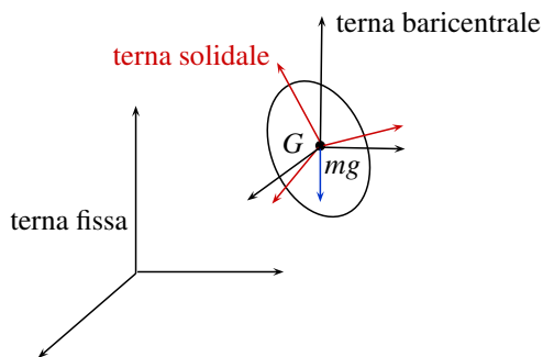
Figura 13.6.1: Rigido in caduta libera
