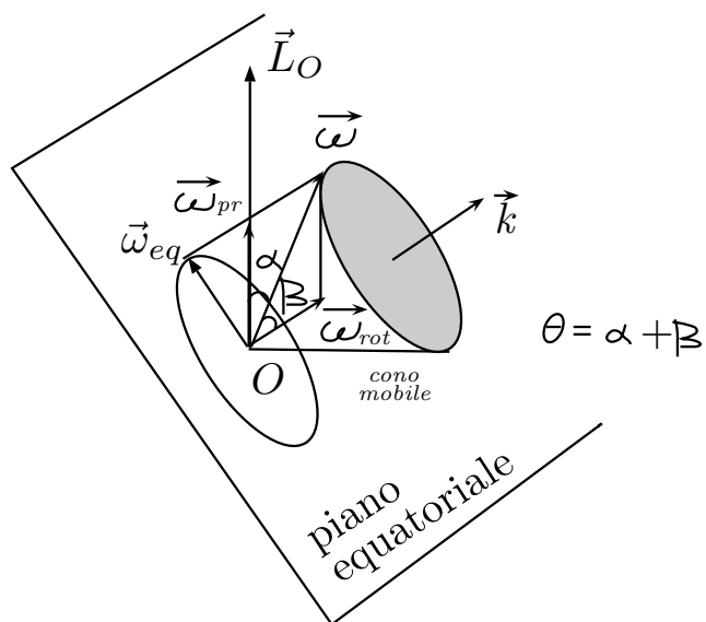
Figura 13.6.4: Cono mobile di Poincaré
