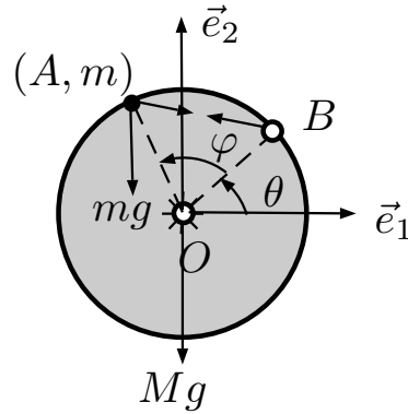
Figura 6.5.1: Diagramma delle forze attive
