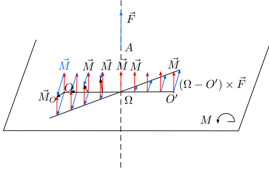
Figura 7.2.3: Campo dei momenti di un torsore: struttura elicoidale
