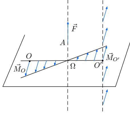
Figura 7.2.1: Campo dei momenti di una singola forza: struttura rotatoria
