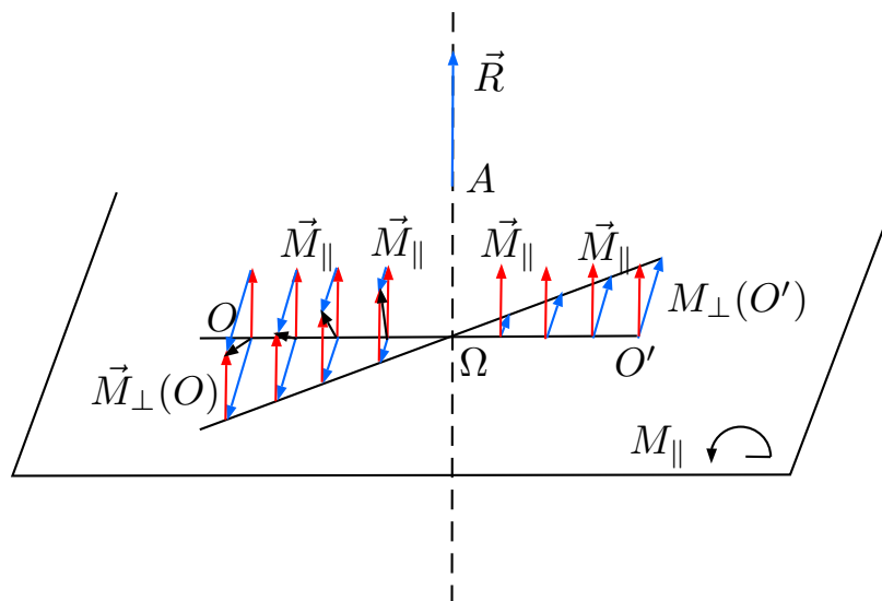
Figura 7.3.1: Asse centrale di un insieme di forze
