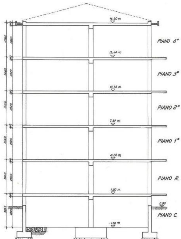
tav. 2 SEZIONE A-A
