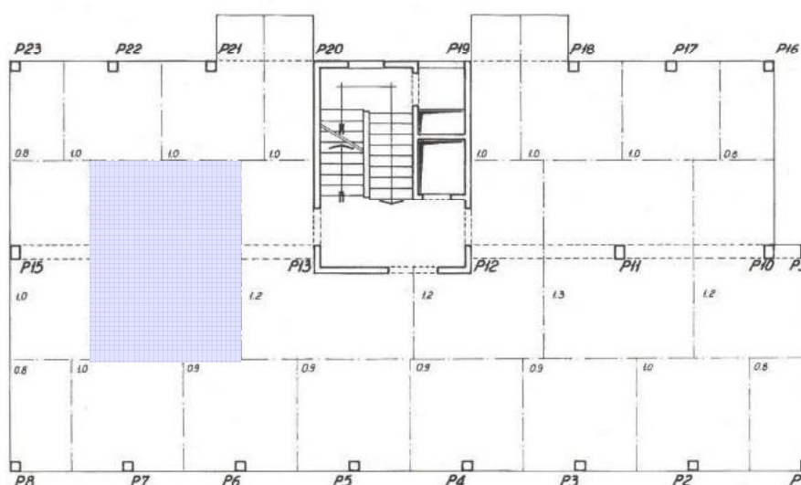
tav. 3 AREE D'INFLUENZA PILASTRI
