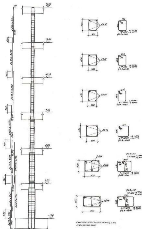
tav. 4 PILASTRO P14
