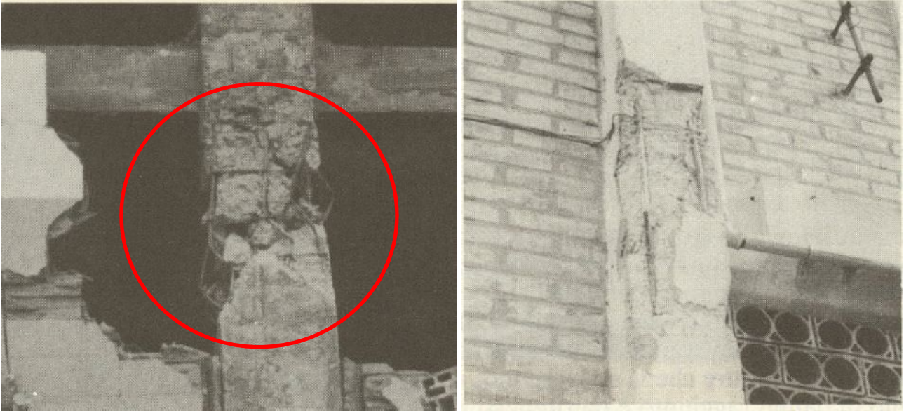
Instabilizzazione barre di armatura compresse per eccessiva spaziatura delle staffe
