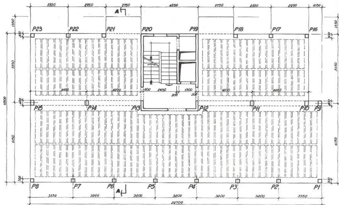
tav. 1 PIANTA PIANO TIPO
