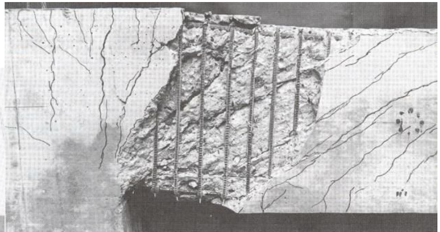
Instabilizzazione barre di armatura compresse per eccessiva spaziatura delle staffe
