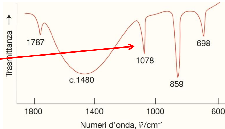
Calcite (esagonale) Aragonite (ortorombica)
