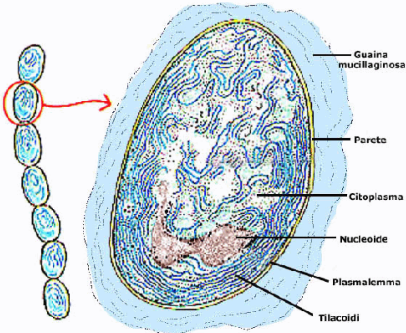
Struttura di una cellula di cianobatterio
