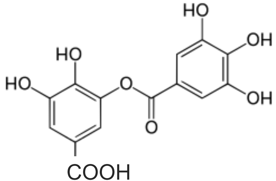
Acido DIGALLICO
