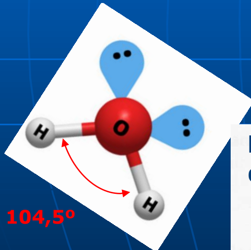
Molecola d'acqua
