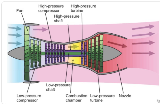
TURBOFAN – Vista in sezione
