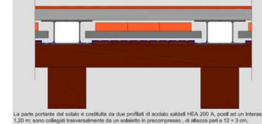
Tipologia S03 Solaio di profilati d'acciaio con solaio latero-cemento
