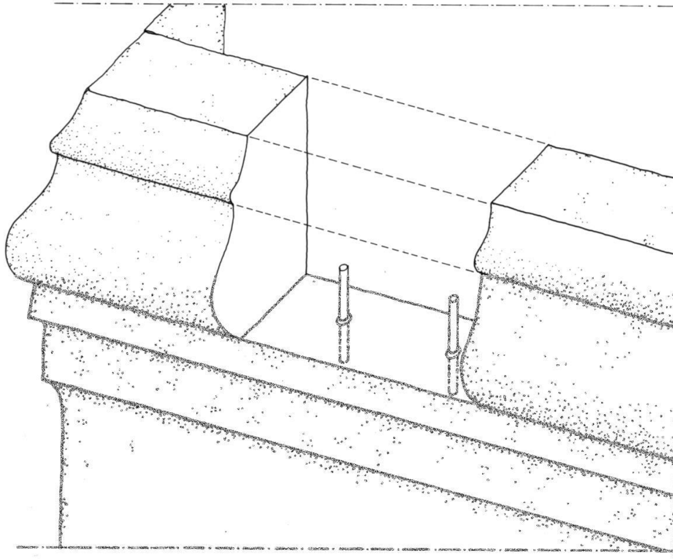
Figura 2 • Tassello per una cornice modanata, inserito dall'alto verso il basso. Il vincolo è realizzato con due perni metallici verticali e con l'impiego di resine epossidiche.
