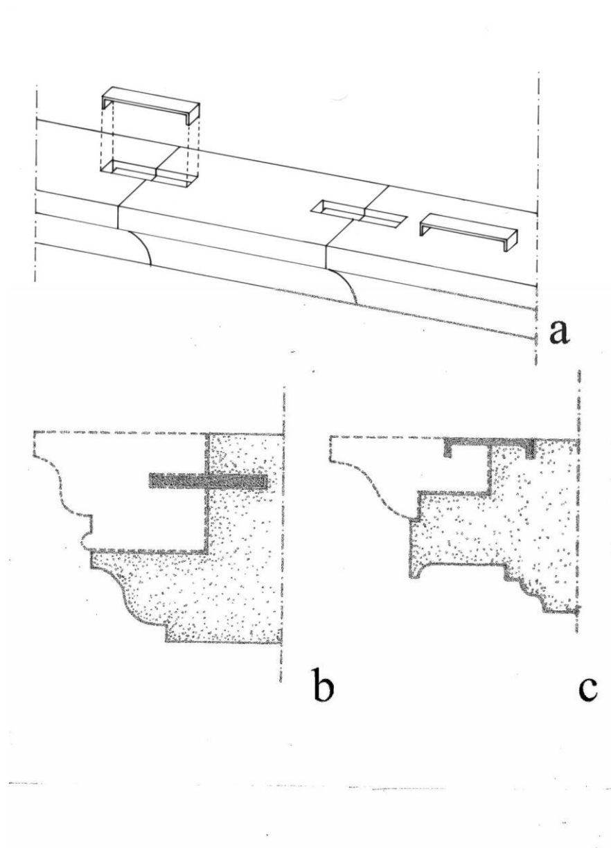
Figura 4 • Tasselli semplici: a) tassello inserito su cornice marcapiano con vincoli metallici (grappe) incassati a livello; b) tassello con tenuta a malta e perno metallico; c) tassello con tenuta a malta e grappa metallica.
