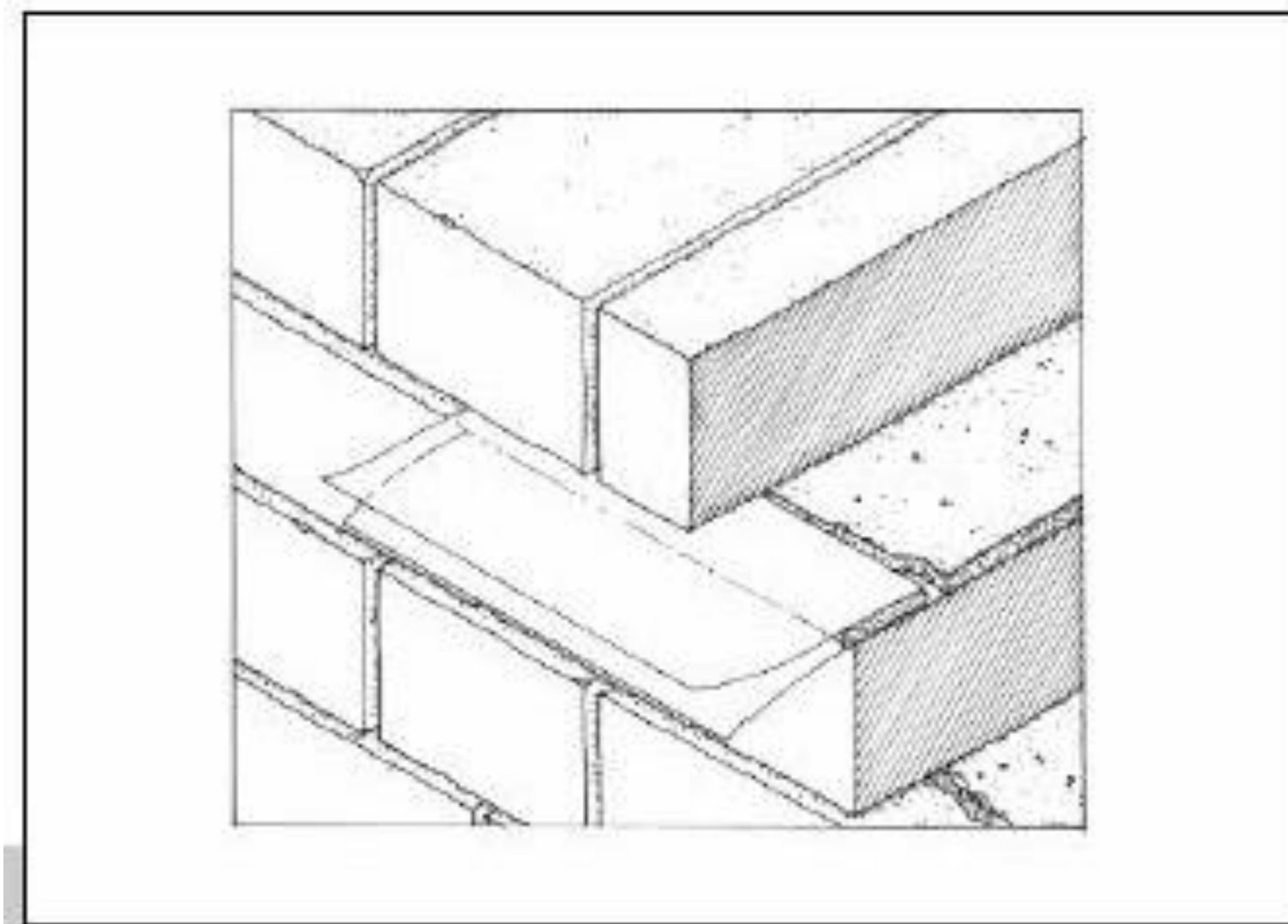
Figura 7 • In funzione della dimensione del giunto e dei materiali che costituiscono il paramento murario, possono essere impiegate diverse procedure. Qui è descritto il sistema detto a sandwich di stucco: due fogli di pellicola plastica contenenti la necessaria quantità di malta sono introdotti nel giunto da risarcire per mezzo di una lama piatta.
