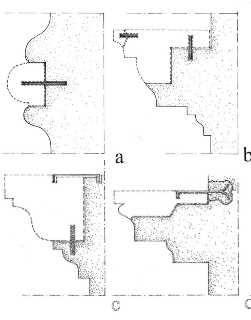
Figura 5 • Tasselli semplici: a) tassello con tenuta a perno metallico; b) rimontaggio di frammenti, con perni metallici di diversa dimensione; c) tassello con tenuta a malta e grappa metallica; d) in questo caso particolare, la grappetta ha, ad un estremo, una testa a squadra e, sull'altro, due lembi divaricati per essere murati.
