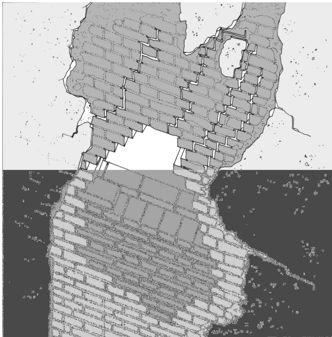
Figura 2 • “Presentazione” dei nuovi pezzi, ovvero loro inserimento provvisorio nella sede prevista, per controllare l’acceptabilità della loro forma e l’effettiva realizzabilità dell’intervento. Posa in opera dei nuovi elementi nelle sedi di inserimento, preparate e pulite nelle fasi precedenti.
