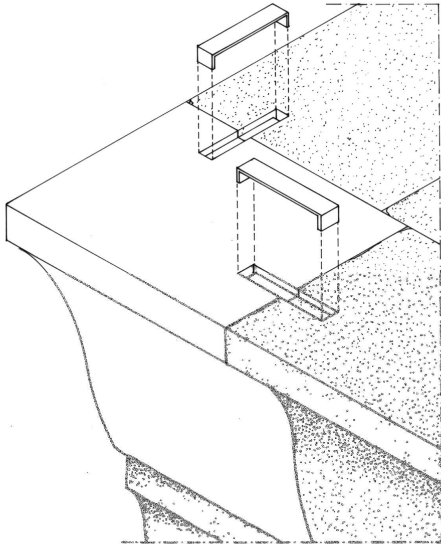
Figura 3 • Tassello di cantone con inserimento di grappe metalliche. Gli alloggi per le grappe sono realizzati con scalpello piano a taglio.
