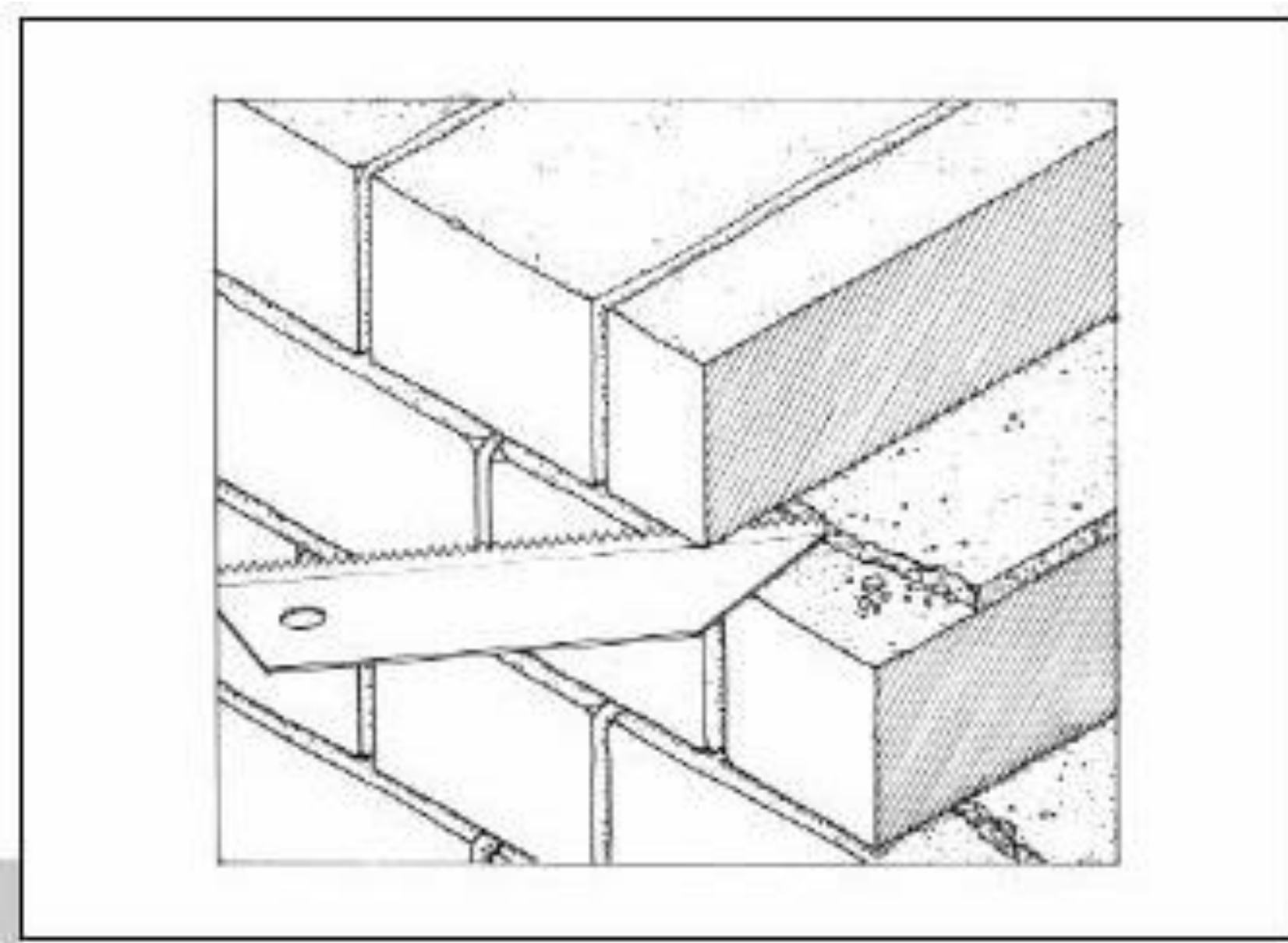
Figura 6 • Per la pulitura dei giunti di dimensioni particolarmente ridotte è necessario intervenire utilizzando lame sottili e dotate di denti.
