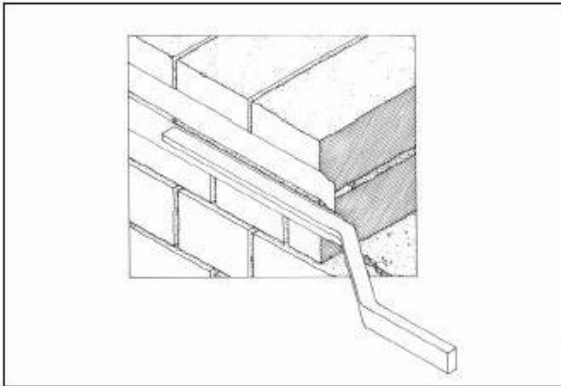
Figura 4 • Stilatura del giunto con un ferro adatto.
