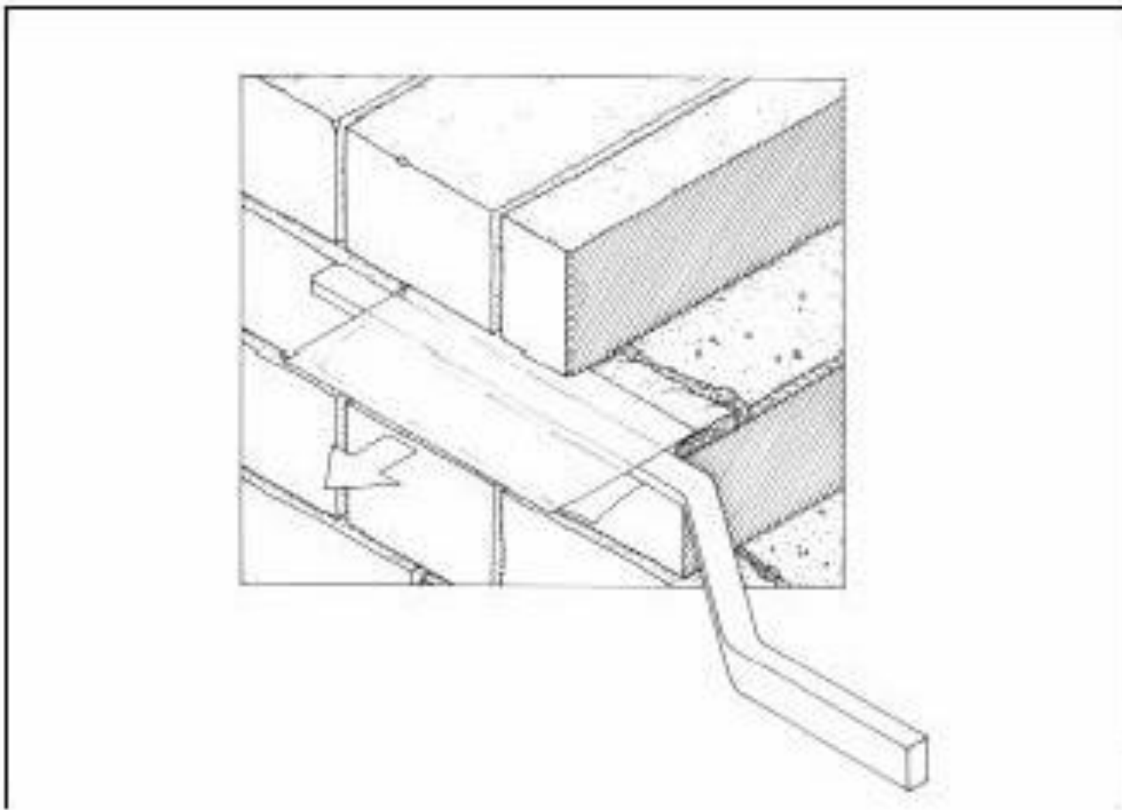
Figura 8 • Contemporaneamente all'operazione di inserimento della malta nel giunto, occorre sfilare i fogli di pellicola plastica. Il materiale in eccesso sarà rimosso con una cazzuola pulita.
