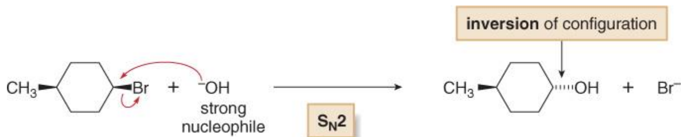
Cis -1-bromo-4-metilcicloesano
