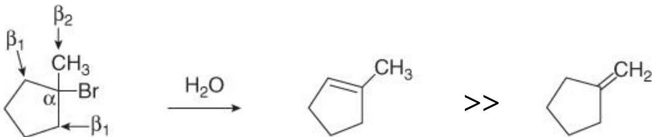
Alchene trisostituito
