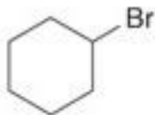
Bromuro 2°
