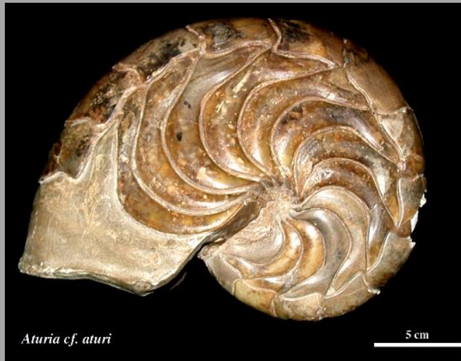
Aturia sp. Miocene, Francia
