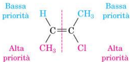
(b) (Z)-2-Cloro-2-butene
