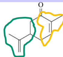
Carvone (olio di menta piperita)
