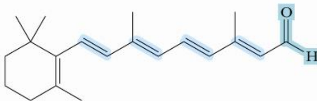
Vitamina A aldeide (retinale)
