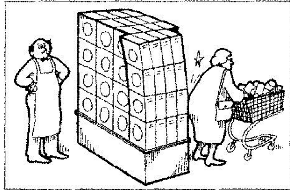
Dislocation Creep
