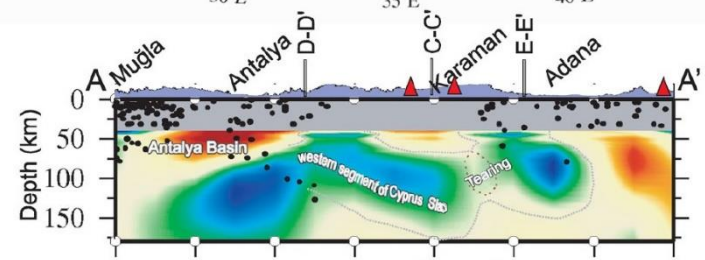
Bakirici et al., 2012, GJI
