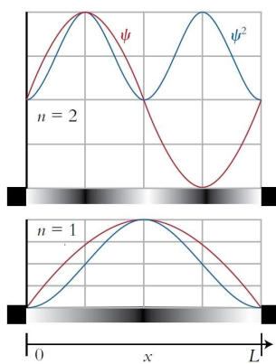
Figura 1C.5 Le due funzioni d'onda ( \psi , rosso) di energia più bassa per la particella nella scatola e le densità ( \psi^2 , blu) corrispondenti. In evidenza anche le densità di probabilità illustrate dal grado di ombreggiatura delle bande sottostanti ciascuna funzione d'onda.
