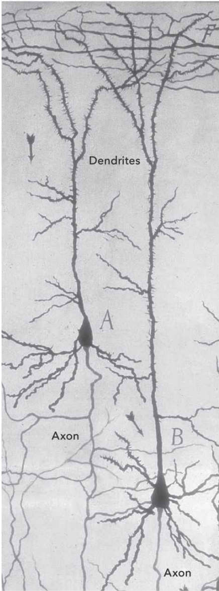
Microcircuits
