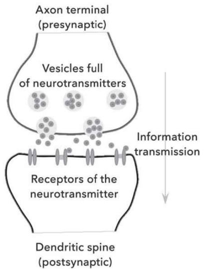
Synapses
