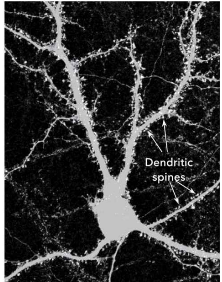
Synapses
