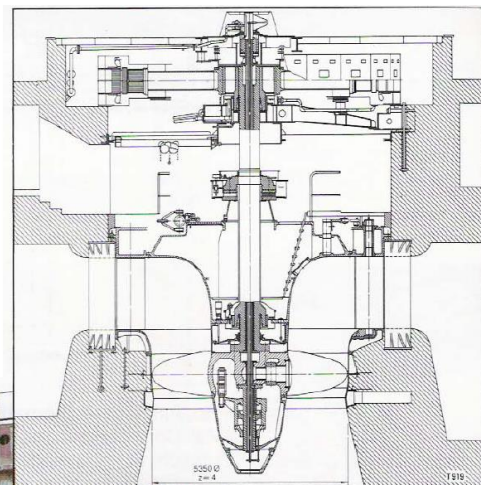
Sezione principale di una turbine a flusso assiale (Kaplan) con caduta utile di 6m, velocità di rotazione 1,3 giri/s, Potenza 6.88 MW e fotografia della girante in officina (Voith).
