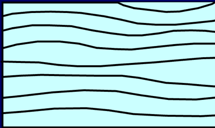
Subparallel
