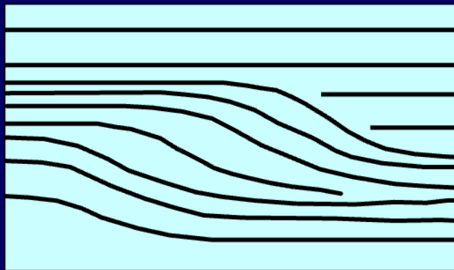
Sigmoid
