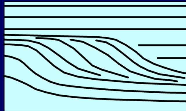
Oblique
