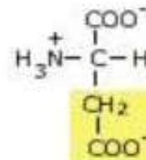
Ac. aspartico
