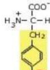
Tirosina
