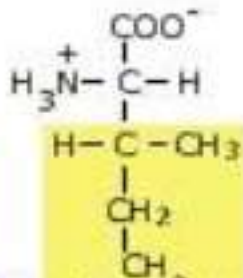
Isoleucina
