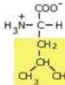
Leucina
