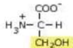
Serina
