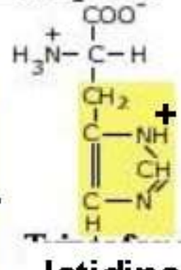
Istidina
