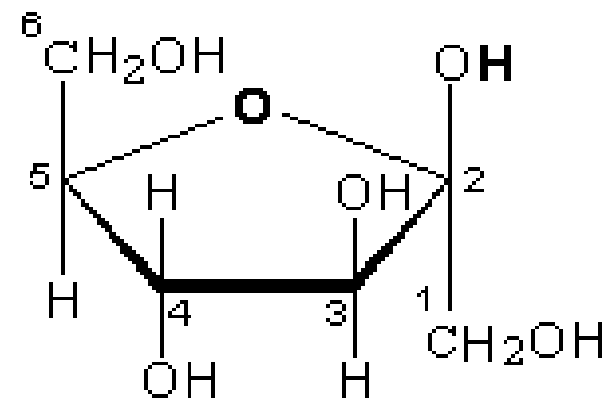
Fruttofuranosio
