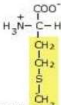
Metionina
