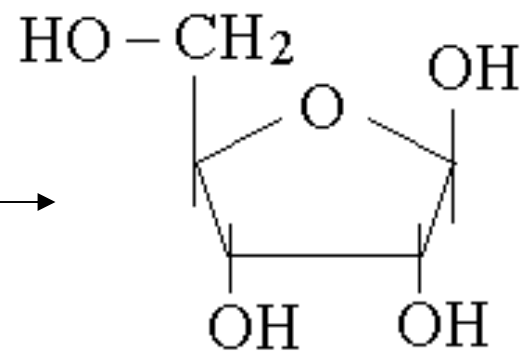
ribosio
