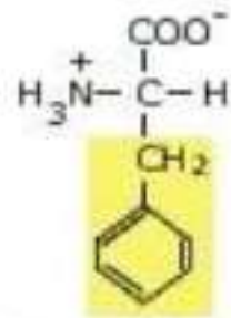
Fenilalanina
