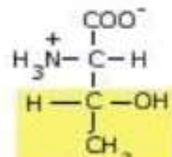
Treonina
