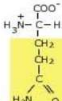
Glutammina
