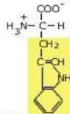
Triptofano
