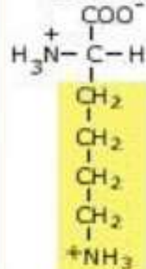
Lisina
