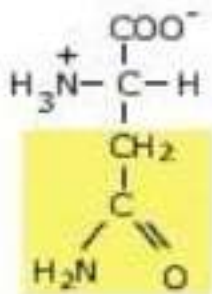
Metionina
