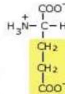
Ac. glutammico
