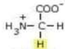
Glicina
