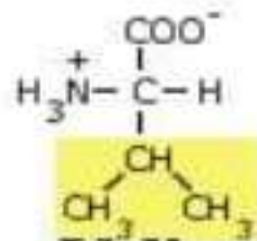
Valina
