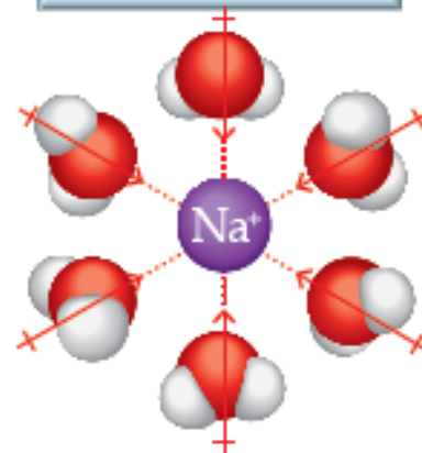
Acqua ( H_2O )
