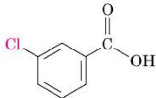
Acido m -clorobenzoico
