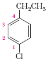
1-Cloro-4-etilbenzene ( p -Cloroetilbenzene)
